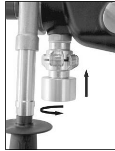
Dispositivo de conexión a un aspirador de polvo
