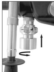
Zařízení pro připojení k odsavači prachu
