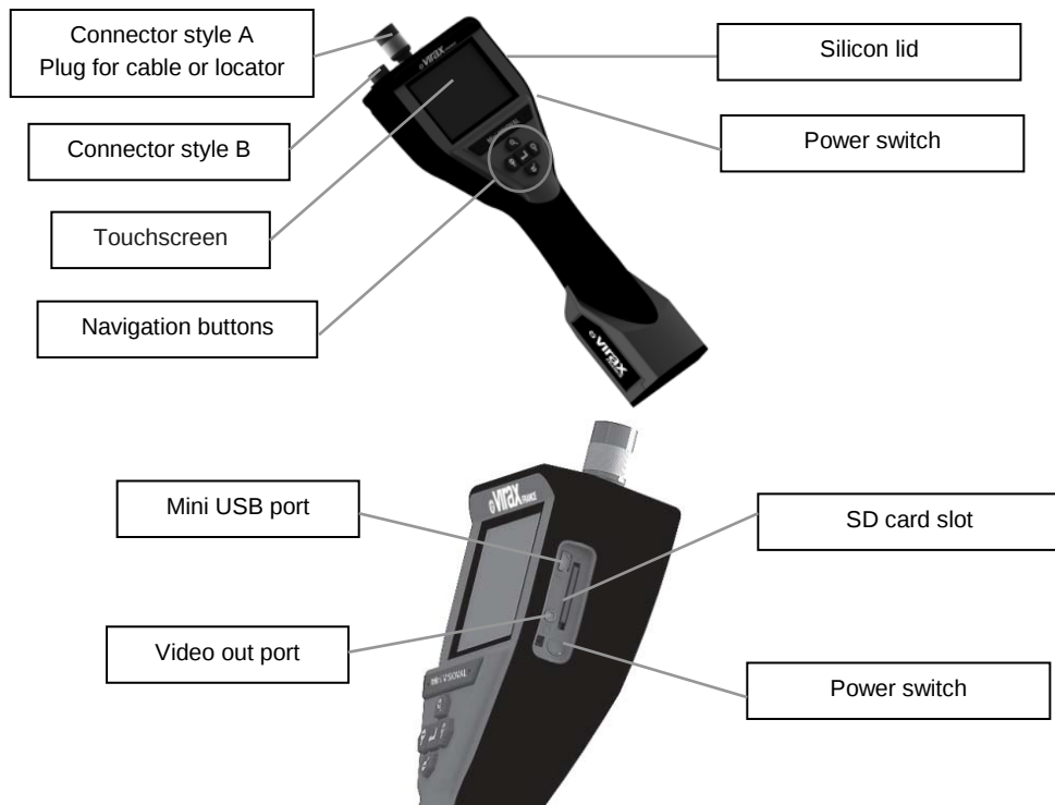
Figure 2 – Mini VISIOVAL
