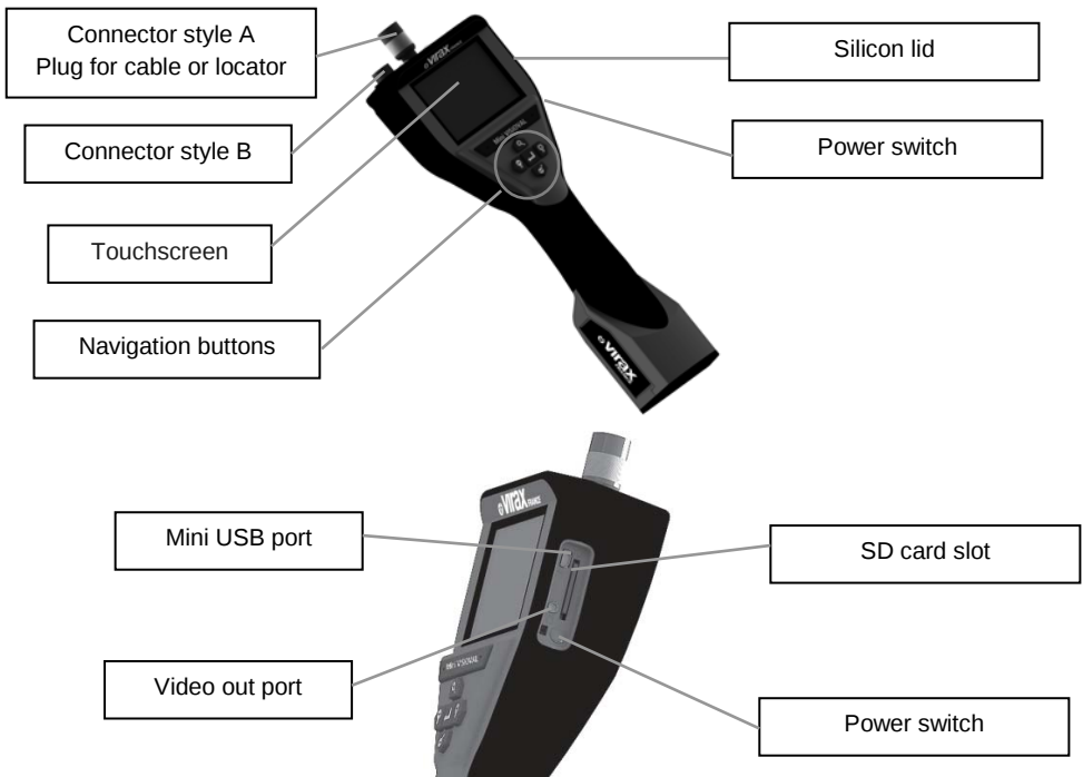
Abb. 2 – Mini VISIOVAL
