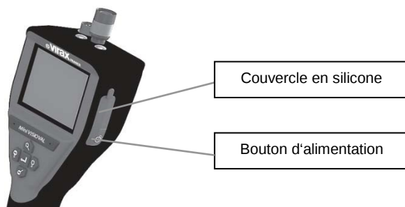
Figure 6 – Couvercle du port et bouton d'alimentation
