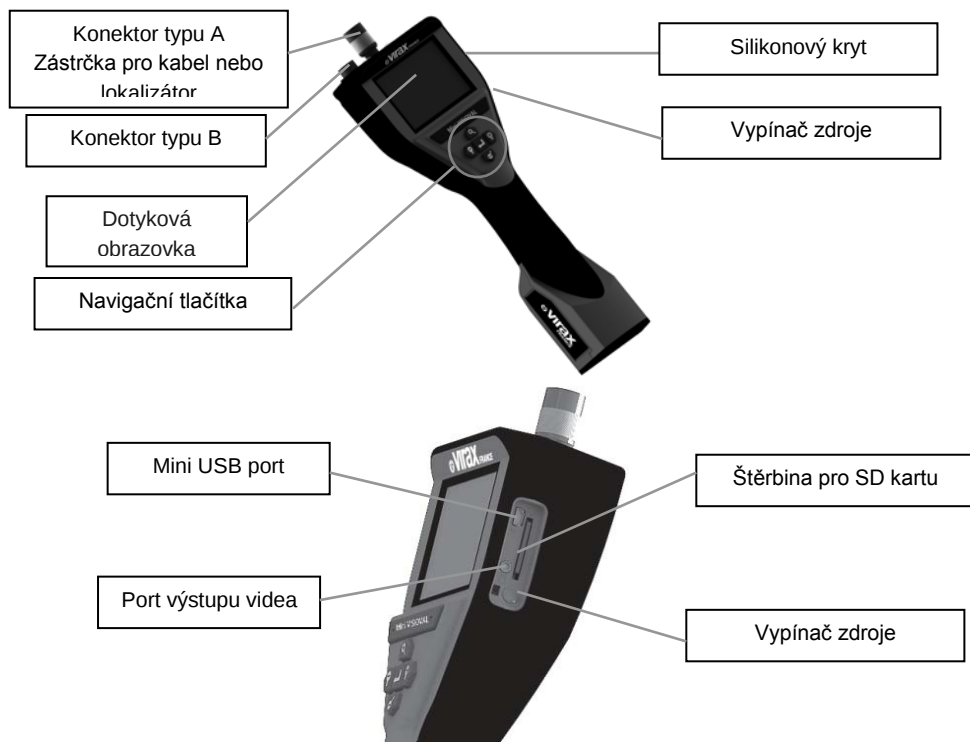
Obrázek 2 – mini VISIOVAL
