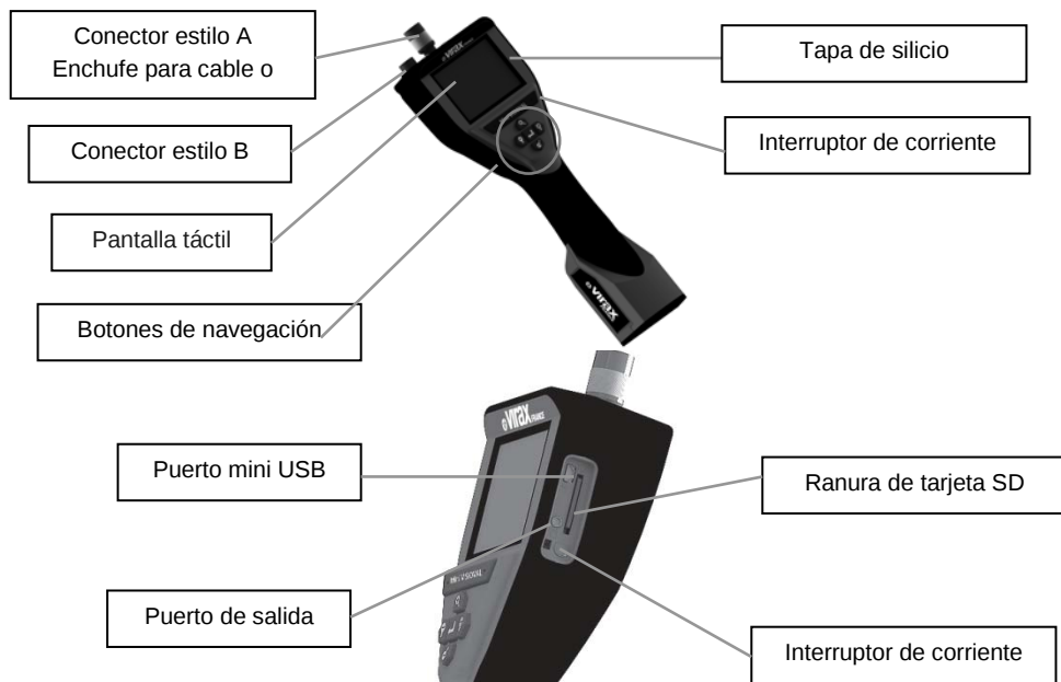
Figura 2 - Mini VISIOVAL
