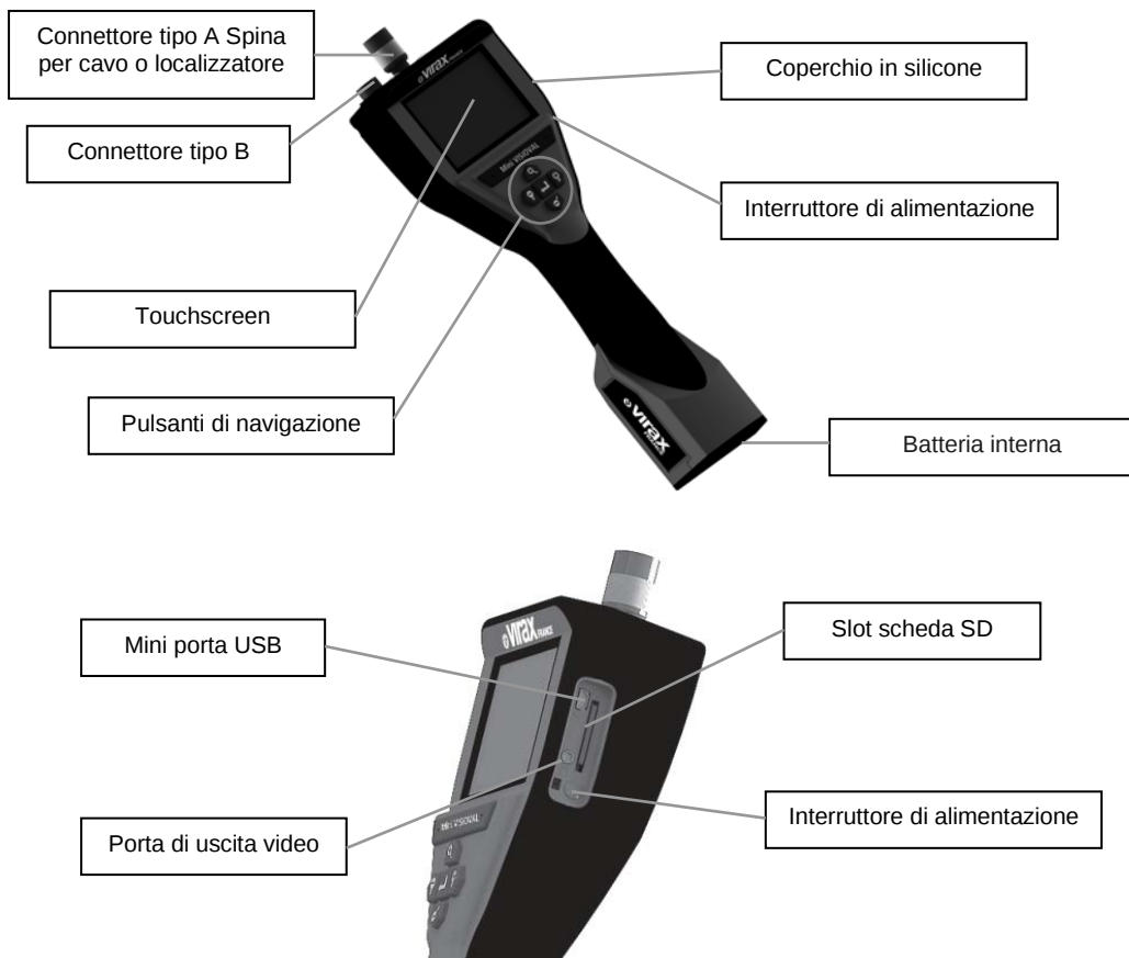
Figura 2 – Mini VISIOVAL
